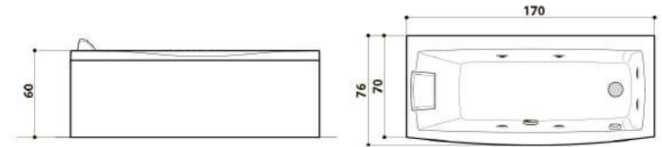
Left hand version view · Abb. Linksausführung
