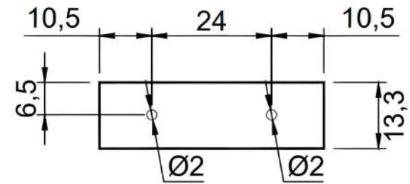
versione da parete wall version
