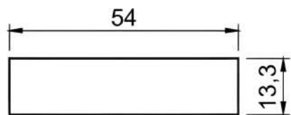
versione soprapiano top mounted version
