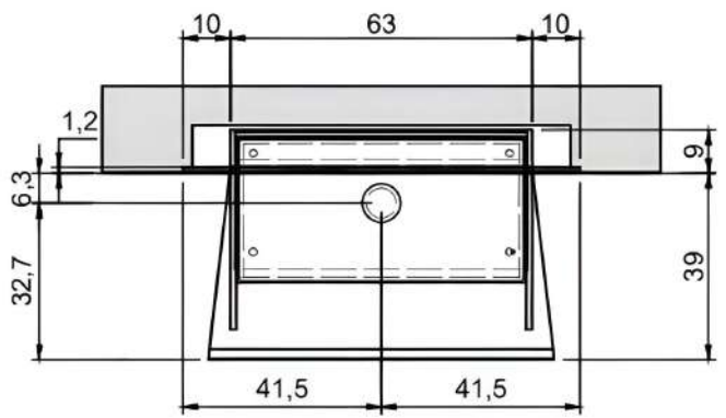
Prospetto frontale Front elevation
