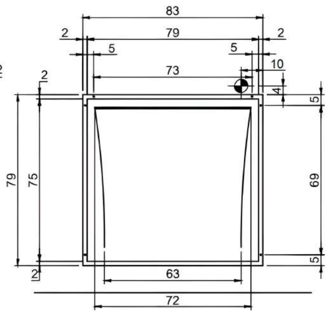
Prospetto frontale Front elevation
