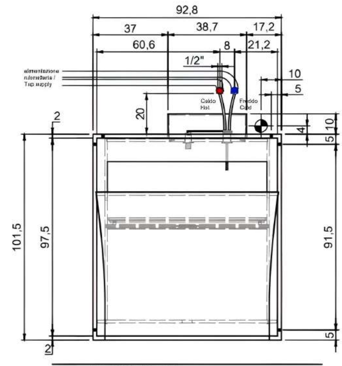
Prospetto frontale Front elevation
