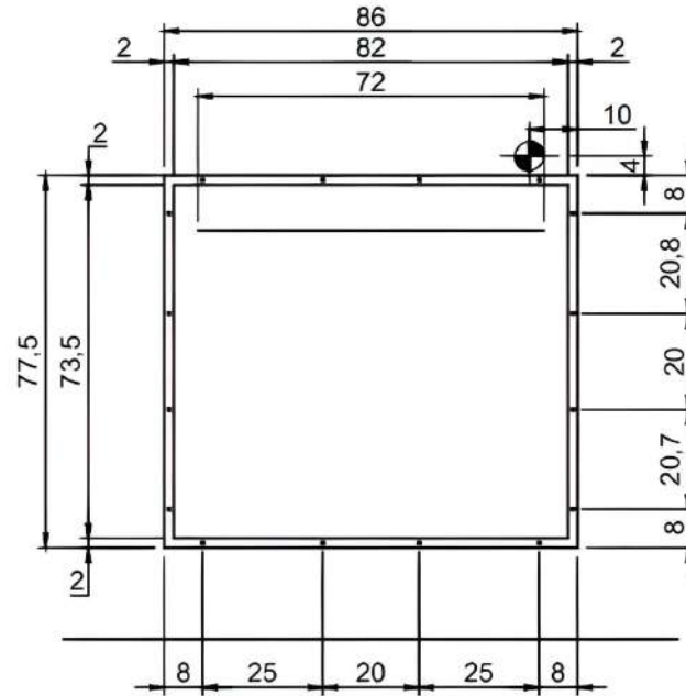
Prospetto frontale Front elevation
