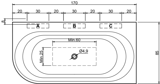
(Vasca decentrata sx o dx ed in basso - versione SX / Off-center bathtub in depth and LH or RH - left version) art. OASI53S peso lordo/gross weight: kg 144 ca peso netto/net weight: kg 119 ca
