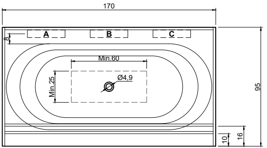
(Vasca centrale / Centered bathtub) art. OASI86M peso lordo/gross weight: kg 204 ca peso netto/net weight: kg 119 ca
