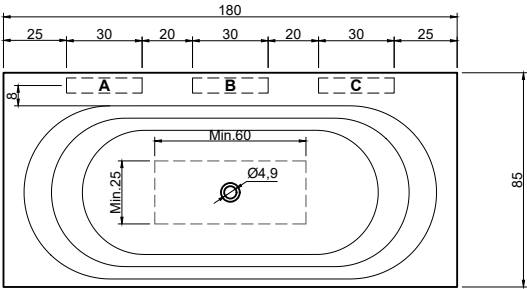
(Vasca decentrata in basso / Off-center bathtub in depth) art. OASI74FC peso lordo/gross weight: kg 149 ca peso netto/net weight: kg 124 ca
