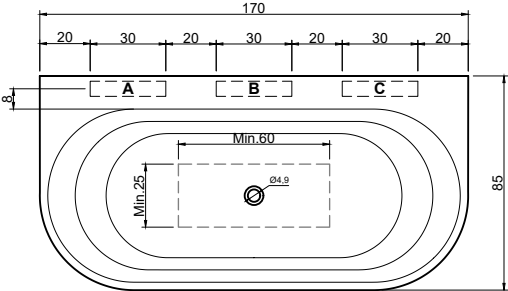
(Vasca decentrata in basso / Off-center bathtub in depth ) art. OASI63 peso lordo/gross weight: kg 144 ca peso netto/net weight: kg 119 ca
