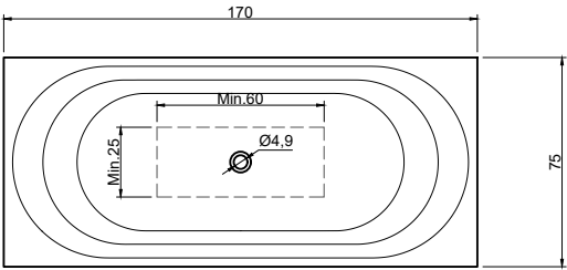
(Vasca centrale / Centered bathtub) art. OASI30 peso lordo/gross weight: kg 85 ca peso netto/net weight: kg 60 ca
