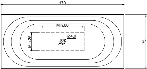
(Vasca centrale / Centered bathtub) art. OASI70 peso lordo/gross weight: kg 138 ca peso netto/net weight: kg 113 ca
