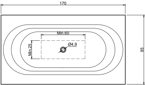
(Vasca centrale / Centered bathtub) art. OASI76M peso lordo/gross weight: kg 150 ca peso netto/net weight: kg 125 ca
