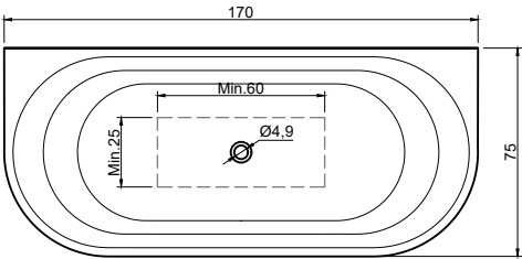
(Vasca centrale / Centered bathtub ) art. OASI60 peso lordo/gross weight: kg 138 ca peso netto/net weight: kg 113 ca
