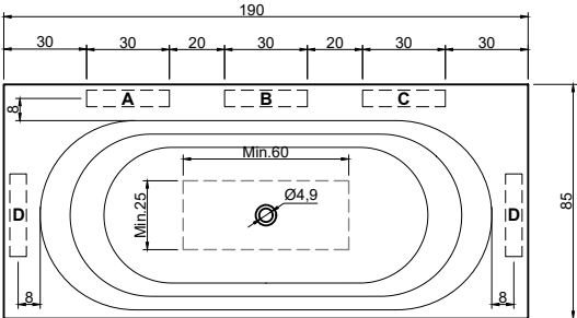
(Vasca decentrata in basso / Off-center bathtub in depth) art. OASI75FC peso lordo/gross weight: kg 153 ca peso netto/net weight: kg 128 ca
