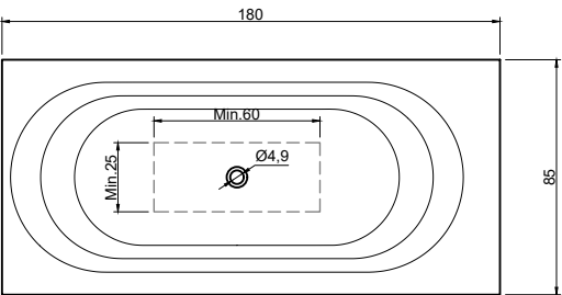
(Vasca decentrata sx o dx - versione sx / Off-center bathtub LH or RH - Left version)
