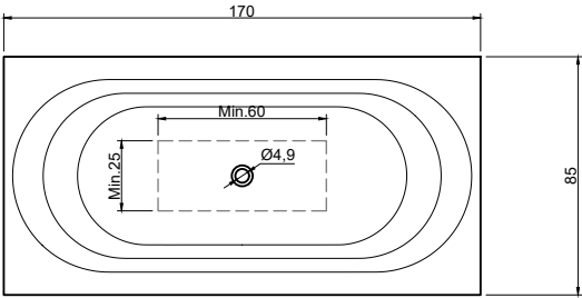
(Vasca centrale / Centered bathtub) art. OASI73M peso lordo/gross weight: kg 204 ca peso netto/net weight: kg 119 ca
