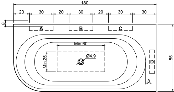
(Vasca decentrata sx o dx ed in basso - versione SX / Off-center bathtub in depth and LH or RH - left version) art. OASI54S peso lordo/gross weight: kg 149 ca peso netto/net weight: kg 124 ca
