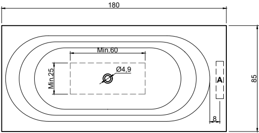
(Vasca decentrata sx o dx - versione sx / Off-center bathtub LH or RH - Left version) art. OASI74MS peso lordo/gross weight: kg 149 ca peso netto/net weight: kg 124 ca
