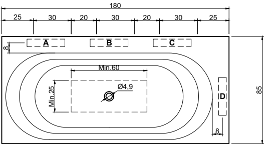
(Vasca decentrata sx o dx - versione sx / Off-center bathtub LH or RH - Left version) art. OASI74FS peso lordo/gross weight: kg 149 ca peso netto/net weight: kg 124 ca
