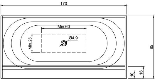
(Vasca centrale / Centered bathtub) art. OASI83M peso lordo/gross weight: kg 204 ca peso netto/net weight: kg 119 ca
