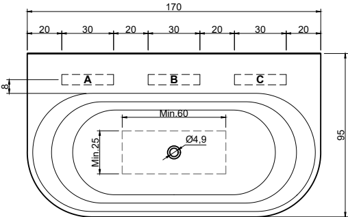
(Vasca decentrata in basso / Off-center bathtub in depth ) art. OASI66 peso lordo/gross weight: kg 150 ca peso netto/net weight: kg 125 ca
