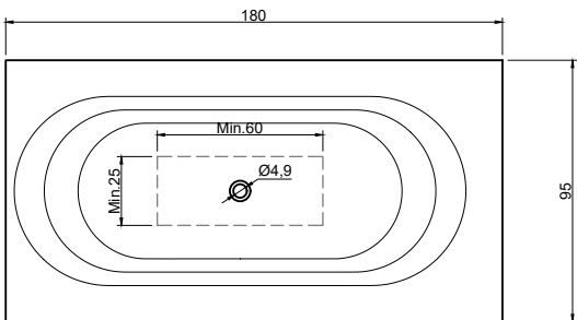
(Vasca decentrata sx o dx - versione SX / Off-center bathtub LH or RH - left version)
