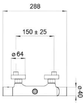
однорычажный для колонны арт. L10173
