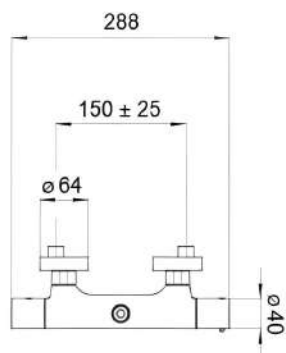
термостатический для колонны арт. L10172
