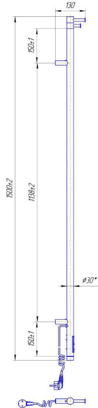
Регулятор 1500x30/130 TR таймер с регулятором
